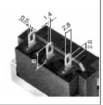
Solder Lug (ON-ON)
