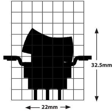
Silhouette (CLD05)
