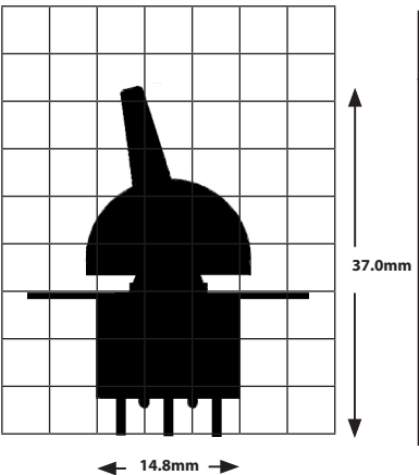
Silhouette (FXED11)
