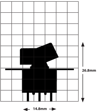
Silhouette (FXED21)
